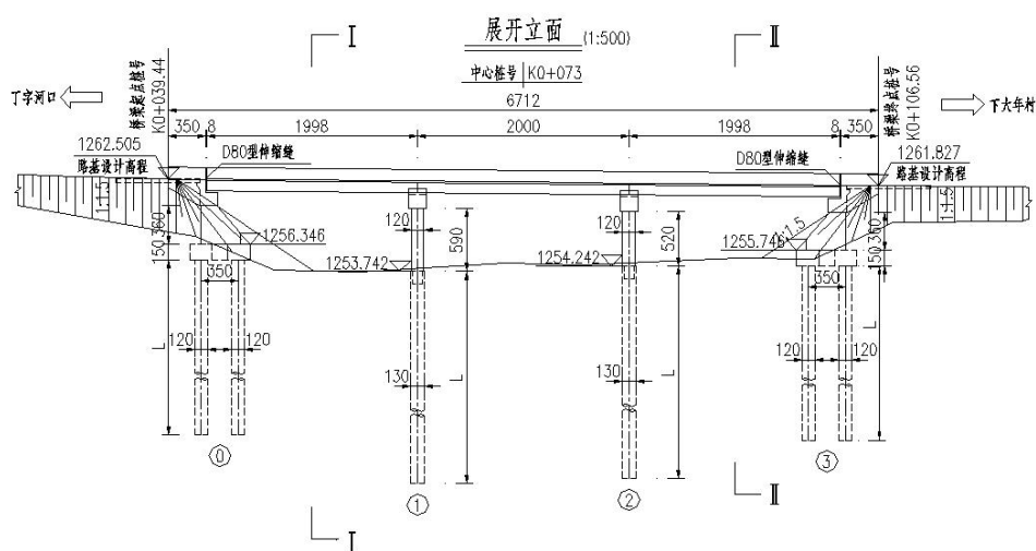
图 2-1 桥梁立面布置图
